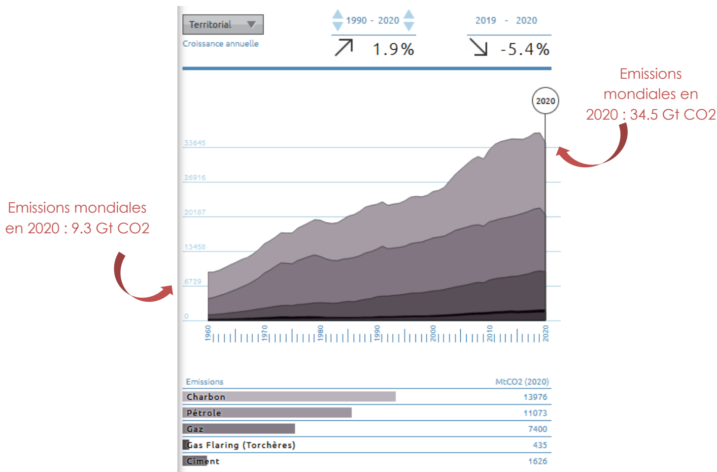
Emissions mondiales de dioxyde de carbone (CO 2 ) liées aux énergies fossiles
