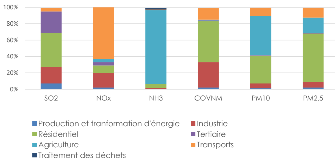
a) La répartition des polluants sur Troyes Champagne Métropole en 2019
