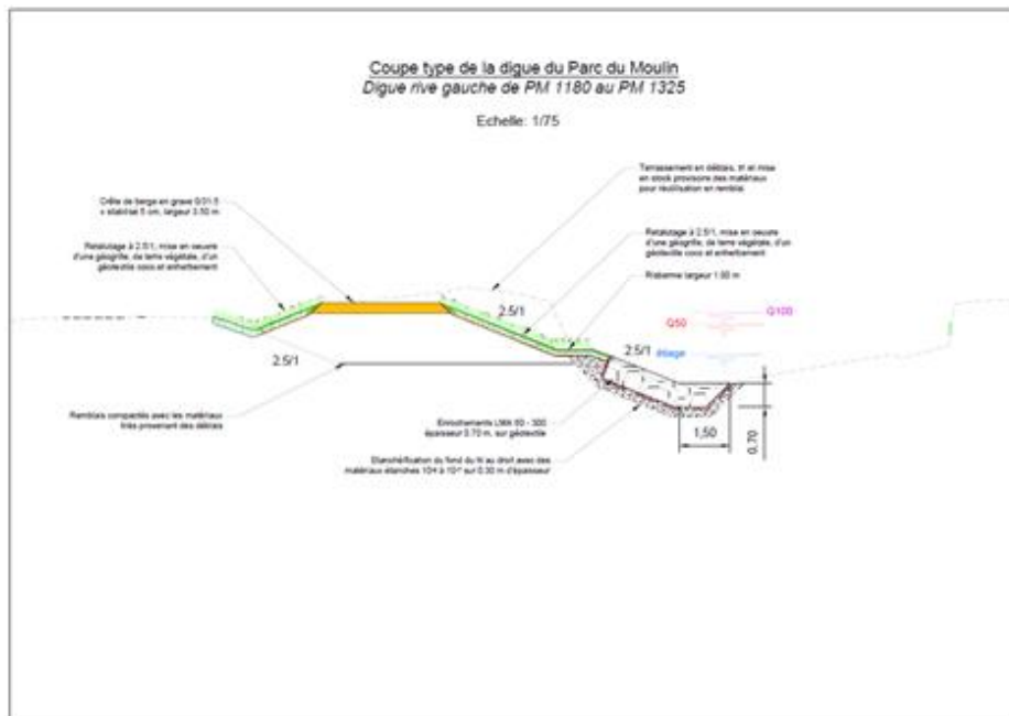
Figure 6 : coupe-type de la digue de Bolloré rive gauche dans le Parc des Moulins
