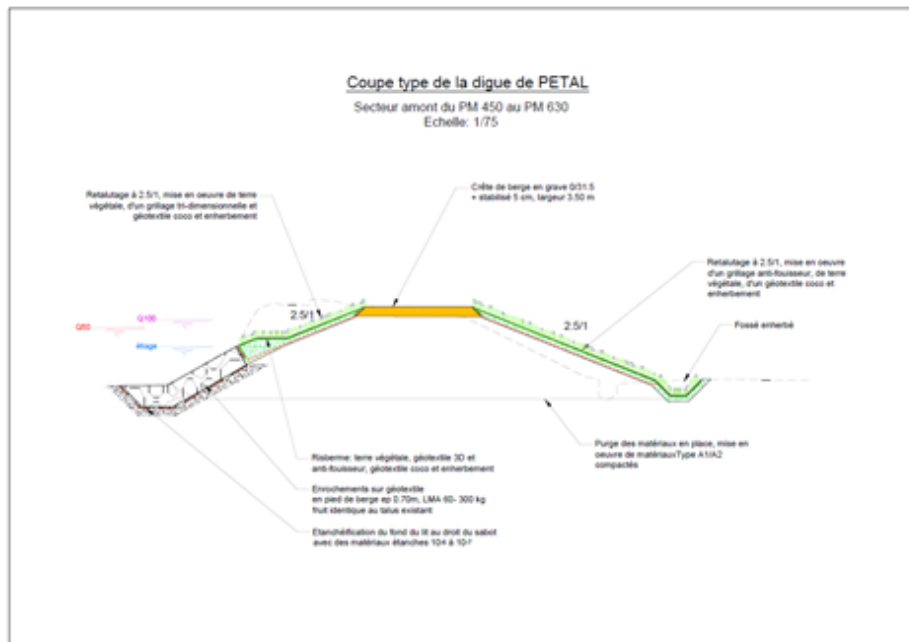
Figure 7 : coupe type de la digue de Pétal sur sa partie amont
