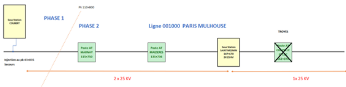
Principe d'alimentation de la phase 2
