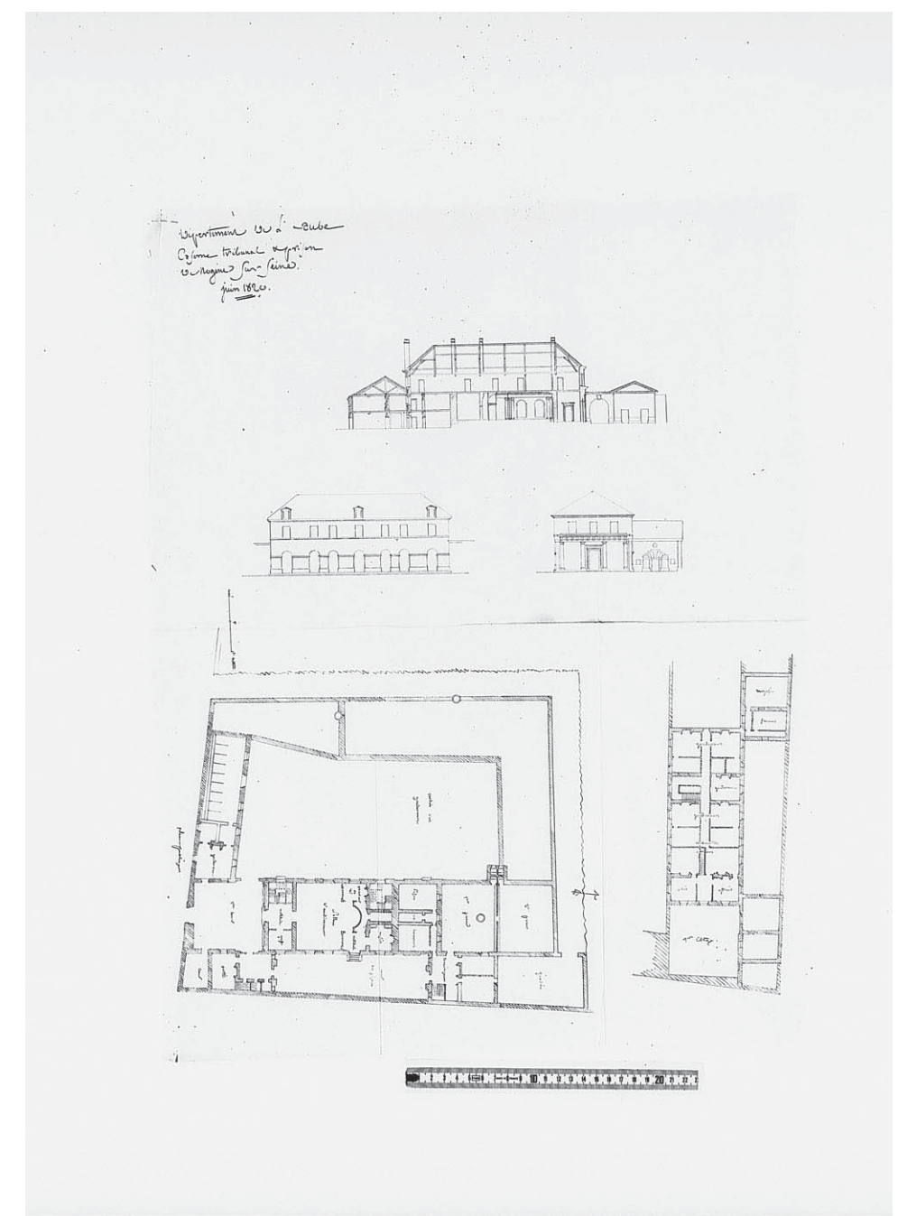
Caserne tribunal prison, calque, Archives Nationales : F/21/1877 ; jaquette 0260, Conseil général des Bâtiments Civils
